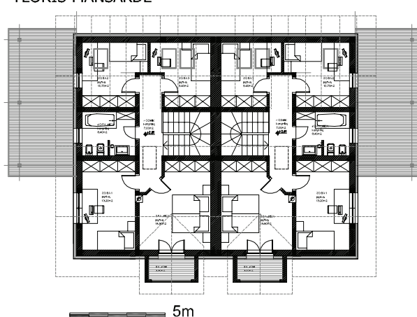
STANOVANJSKI DVOJČEK - OBJEKT B,D TLORIS MANSARDE
