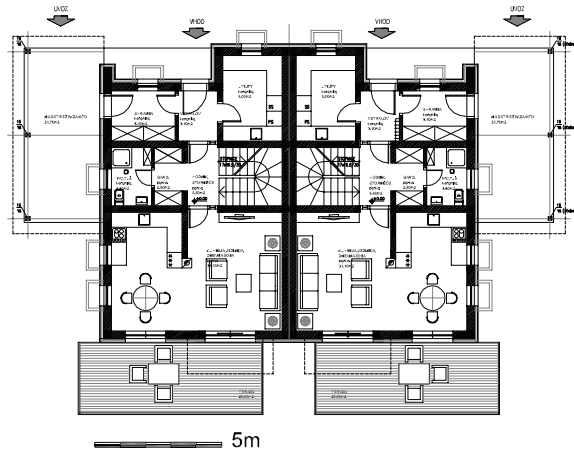
STANOVANJSKI DVOJČEK - OBJEKT B,D TLORIS PRITLIČJA
