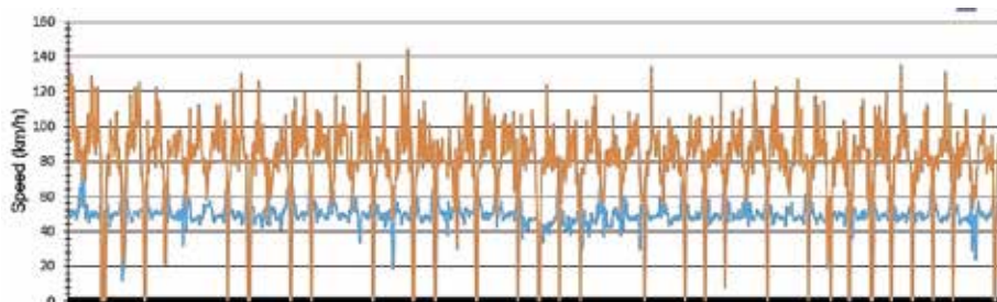
Graf meritev hitrosti v obe smeri s prikazovalnika pri Cvetu gora za mesec julij 2022. Oranžni graf prikazuje izmerjene hitrosti v obe smeri za cel mesec julij, modri graf pa povprečno hitrost. Razvidno je, da so bile hitrosti nad 100 km/h skoraj vsakodnevno prisotne. / Foto: arhiv SPV Jezersko
