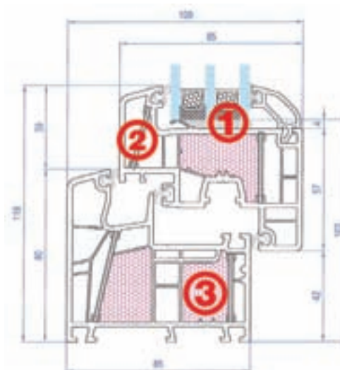
Prerez profila AJM 8000 energeto
