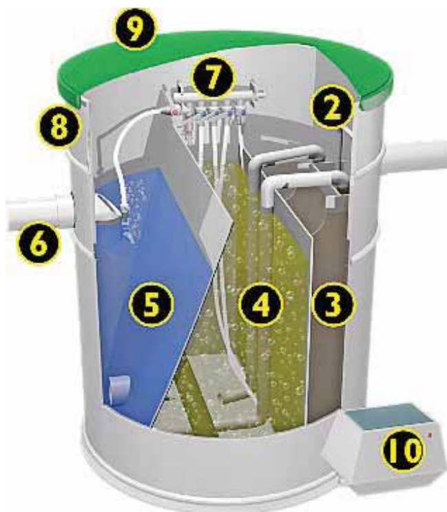
Grafični prikaz delovanja biološke čistilne naprave.
