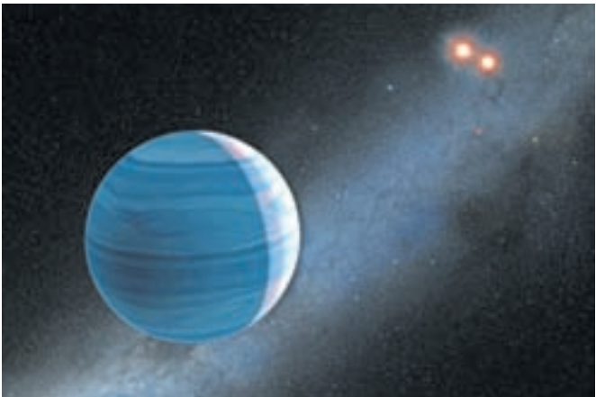
Umetniška podoba eksoplaneta, ki dejansko obstaja in kroži okrog dveh zvezd v osončju OGLE-2007-BLG-349, to pa je od nas oddaljeno 8000 svetlobnih let. / Foto: Wikipedija
