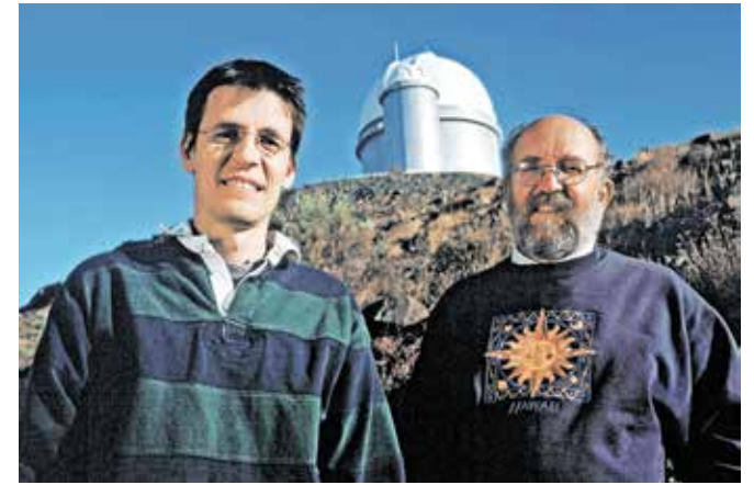
Švicarska astrofizika in Nobelova sonagrajenca Didier Queloz in Michel Mayor pred teleskopom La Silla v Čilu, ki velja za »lovca« na eksoplanete / Foto: Wikipedia
