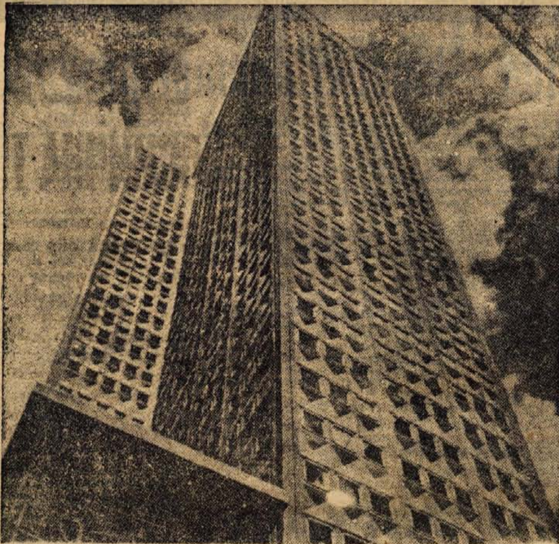
V Pittsburgu (ZDA), svetovnem središču kovinske industrije, so zgradili prvi nebotalnik iz aluminija. Nebotalnik je velilkanska zgradba, ki ima 42 nadstropij in je 123 m visoka. Samo okostje te »aluminijaste hiše« je iz jekla. Vse ostalo je zgrajeno iz aluminija, stekla, kavčuka in iz plastičnih mas. — Prvi aluminijasti nebotalnik so zgradili v kratkem času, saj gradnja ni trajala več kot 6 mesecev
