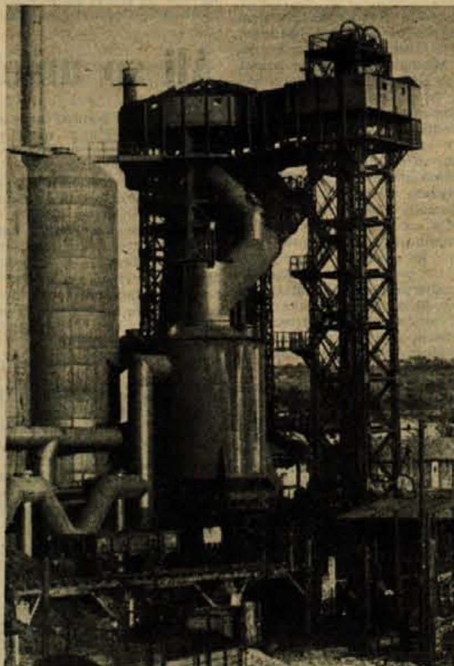
En izmed plavžev v Škednju — pri morju.
