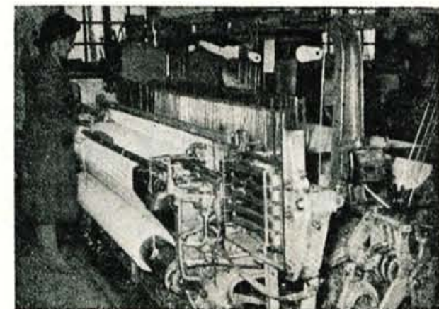
Tkalni stroj s katerim izdelujejo blago od kamgarna do odej
