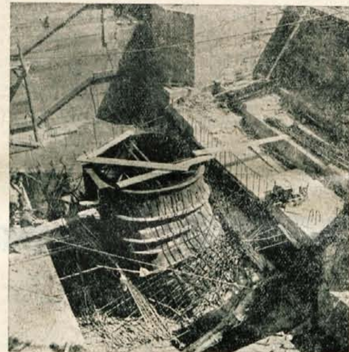
Slika prikazuje jekleno oblogo in armaturo za sesalno cev. Nad njo so kasneje zabetonirali spiralo in montirali turbino
