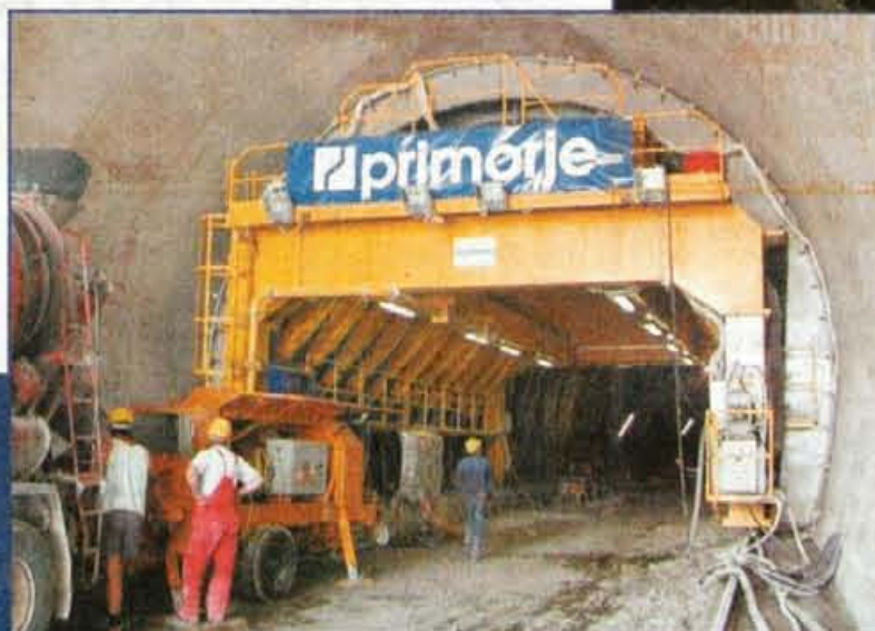
Izdelava betonske obloge s pomočjo posebnega opaža v predoru Kastelec
