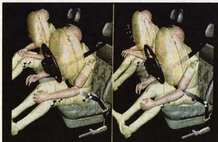
Varnostna zračna vreča se pri trčenjih z manjšo hitrostjo sproži do prve stopnje, pri hujših pa v celoti. Delovanje dvostopenjskih generatorjev nadzira računalnik.
