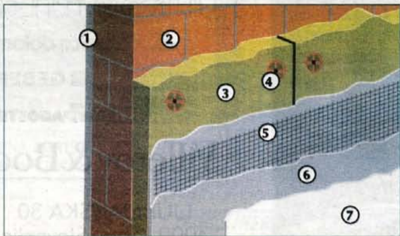
1 - notranji omet; 2 - zid; 3 - TERVOL FPPTL; 4 - pritrdilna sidra; 5 - sloj gradbenega lepila s stekleno armirano mrežico; 6 - drugi sloj gradbenega lepila;
