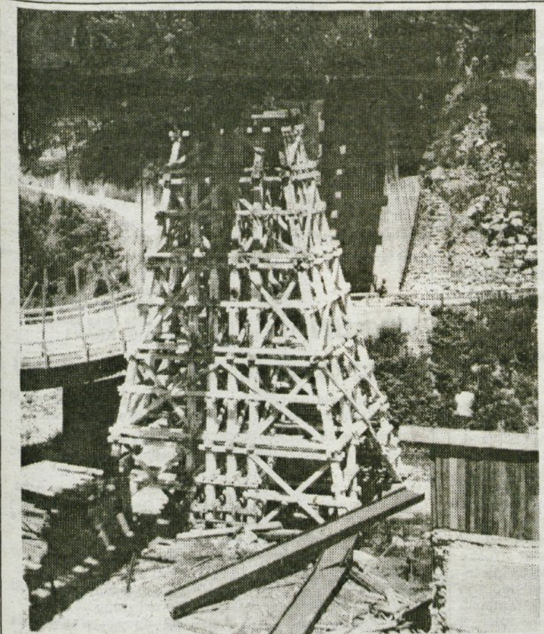
Obnova železniškega mostu pri Žirovnici
