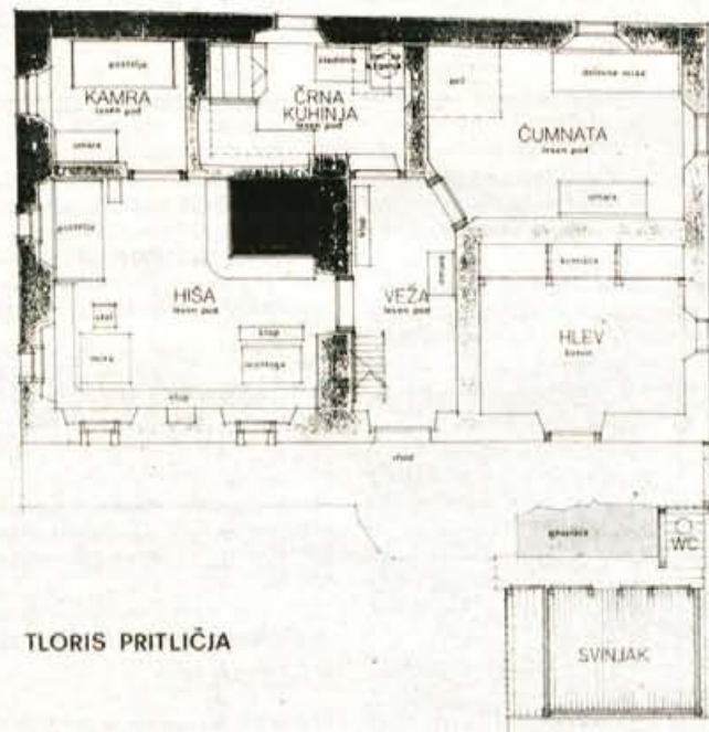
Tloris pritličja Špelčnikove hiše, arh. dokumentacija stud. arh. M. Vojnovič, 1974, Arhiv GM
