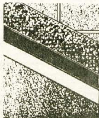
opečni zid Kombi S plošče rabična mrežica cementni obrtsp podlaga na malta zidna omet
