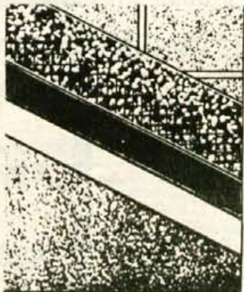
opečni zid KOMBI S plošče rabić mrežica cementni omet pocinkana malta zlatim omet
