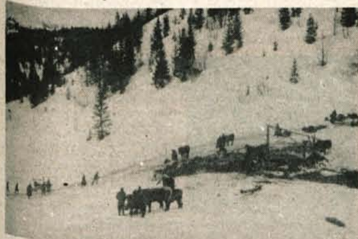
Slika prikazuje zgornjo pogonsko postajo partizanske tovarne žičnice na Koširjevšu. Desno je vitel, ki ga obrača konj. Na levi strani voziček nosilnosti do 250 kg, ki prevaža dele topa po uničenju domobranske postojanke pri Sv. Križu. Žičnica je bila pravo partizansko inovatorstvo. Imela je leseno podporje, nosilno in vlečno vrv, ki jo je vprežna živina navijala na vreteno, za pogon je bil uporabljen vitel.
