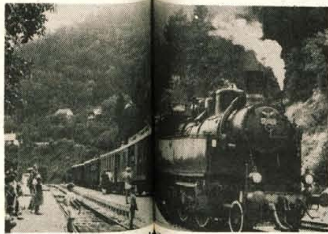
Muzejski vlak z 12 metrov dolgim lokomotivo, ki je težka 54 ton in lahko doseže največjo hitrost 45 kilometrov na uro. — Foto: F. Perdan
