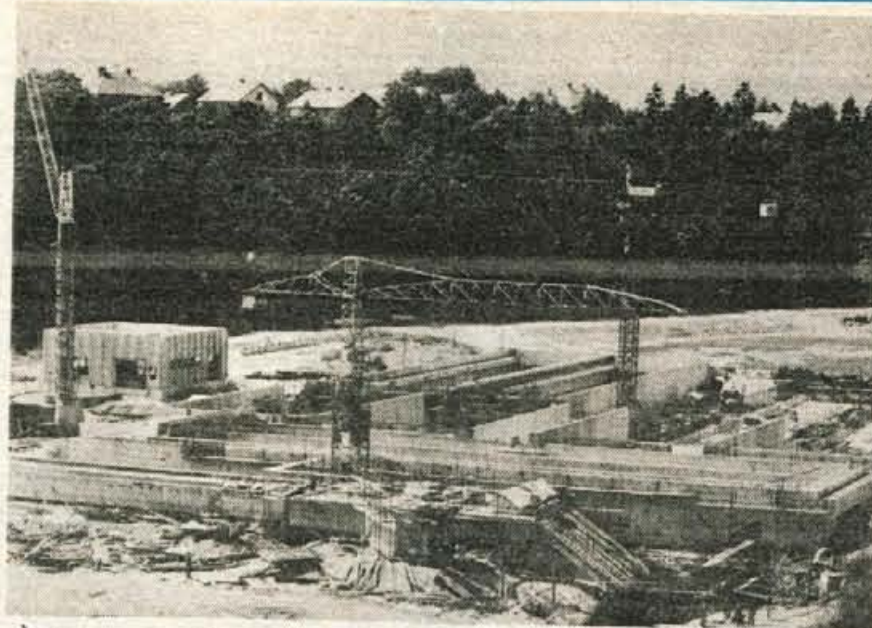
Objekta za predčiščenje in mehansko čiščenje v čistilni napravi sta že gotova. Ostali objekti pa bodo po zagotovljenih izvajalci zgrajeni za poskusno obratovanje do februarja prihodnje leto. Investitorski inženiring in gradbeni nadzor ima Projektivno podjetje Kranj.
