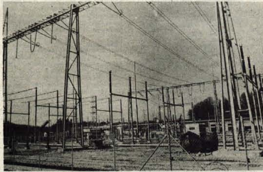
Gradbena dela na razdelilni transformatorski postaji Okroglo gredo h kraju. Postavili so že 400-in 110-kilovoltne zbiralnice s prečnimi povezavami, položen je zemeljski kabel do postaje v Naklem in montiran energetski transformator. Oprema iz kreditu IBRD je dobavljena, izgradnja bo tako najbolj odvisna od dobav preostale opreme. Foto: L. Mencinger
