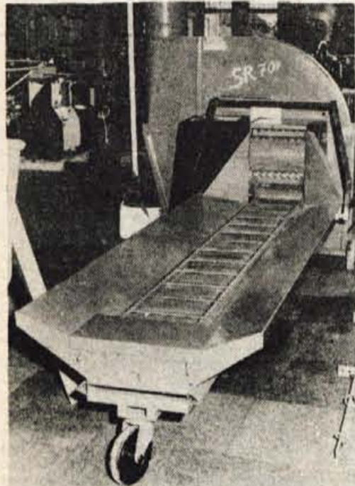
Novo na našem tržišču je domača siloreznica, ki z uporabnostjo, zmogljivostjo ter izvedbo ne zaostaja za tovrstnimi izdelki najbolj znanih inozemskih proizvajalcev.
