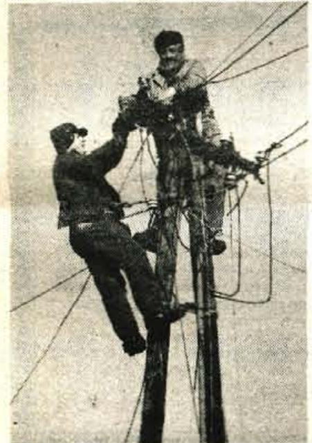
Streha RTP Radovljica se je zrušila na 110-kilovoltno stikališče. Tudi na terenu so popravila terjala od delavcev Elektro Gorenjske veliko naporov.
