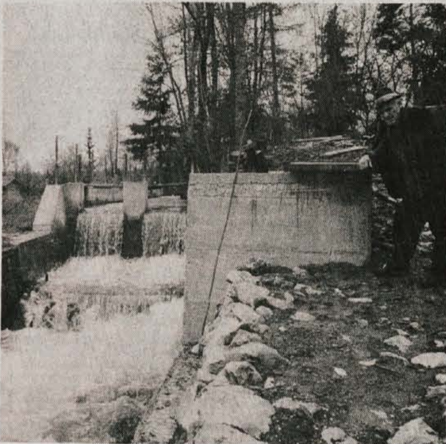
Sr. Bela — Pri Kračmanu, ob rojstni hiši Matije Valjavca, so Belo zajeli in del vode speljali po ceveh do nekaj deset metrov postavljene male elektrarne z močjo do 15 kilovatov. — Foto: L. M.
