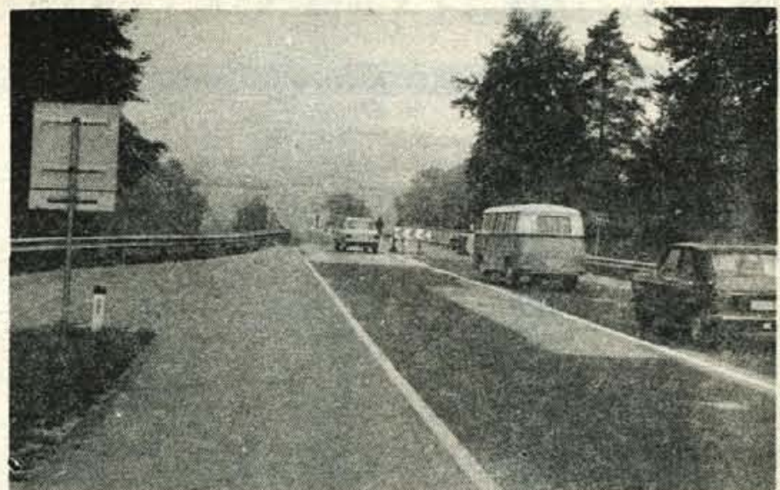
Obnovitvena dela na magistrali - Od viadukta na Peračiči do odcepa ceste proti Trziču v teh dneh potekajo obnovitvena dela na gorenjski magistrali. Na viaduktih polagajo delavci nov asfalt, gradnjo na cesti pa so z znaki dobro označili in vožnjo mimo gradbišča uravnavajo tudi semaforji. Promet kljub delom zato poteka brez večjih zastojev. - Foto: D. Sedej
