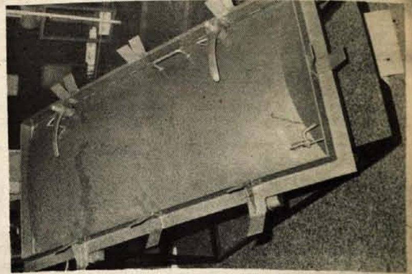
»Kovinarska« Krško proizvaja v sodelovanju s svojimi kooperanti in dobavlja kompletno opremo za zaklonišča, ki je atestirana pri pristojnih institucijah. Med drugim predstavlja na sejmu tudi protidarna in hermetična vrata za zaklonišče in ventilacijsko napravo, ki poleg osnovne namembnosti omogoča v mirnodobnih razmerah uporabljanje zaklonišča tudi za druge namene.
