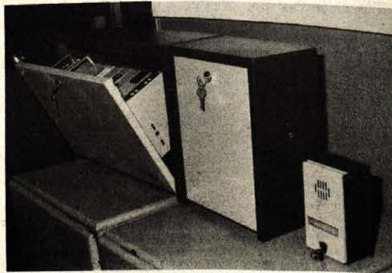
PRÓTIVLOMNA CENTRALA je sabotažno zaščitena in ima trajno kodo za postavljanje programa (dan, noč). Uporablja se vzporedno z javljalniki vloma.
