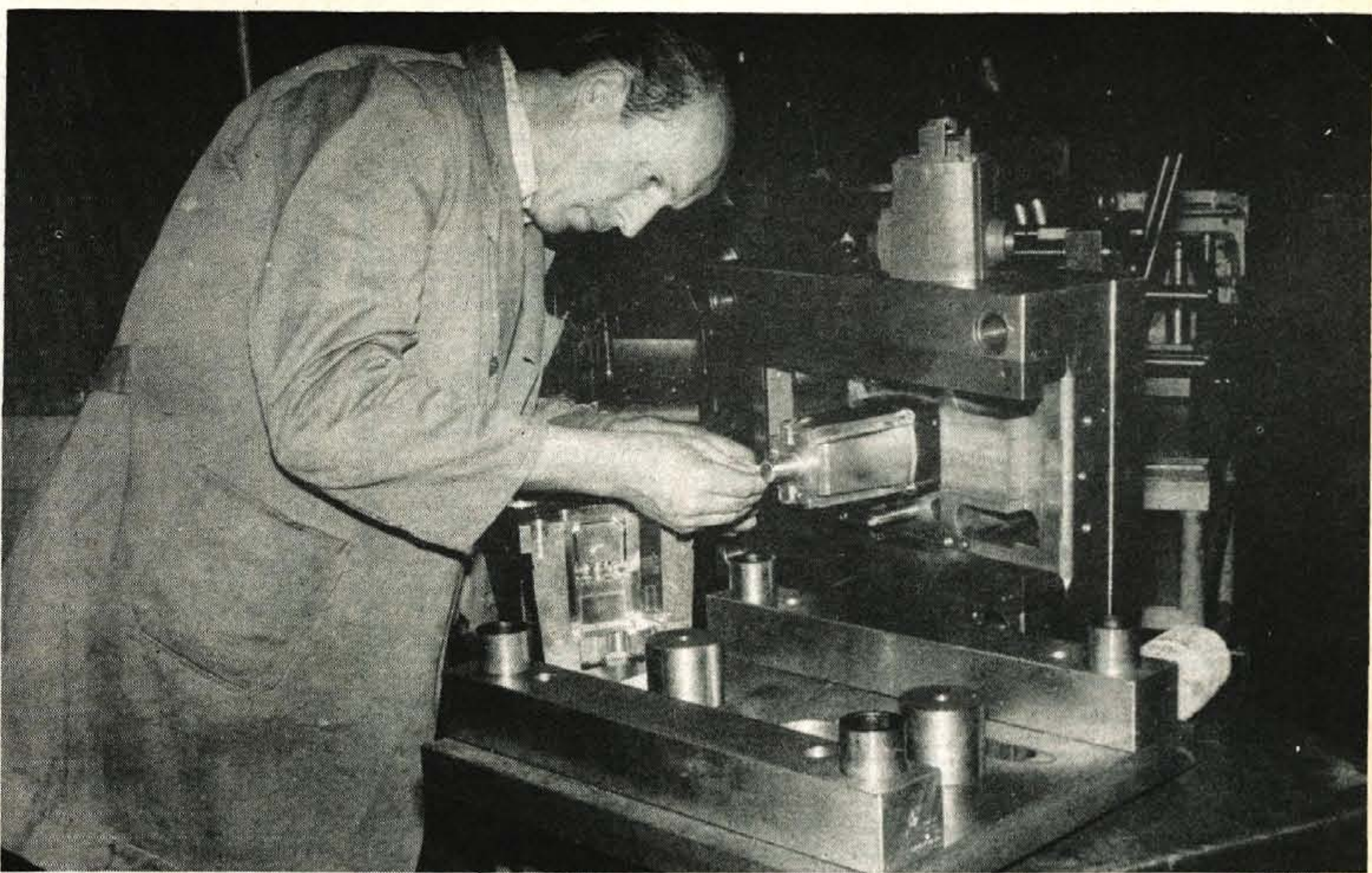
Ročna obdelava orodja za predelavo termostatov
