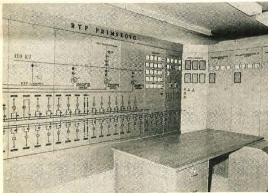
Komandna plošča 10 in 20 kV stikališča nove razdelilne postaje na Primskovem
