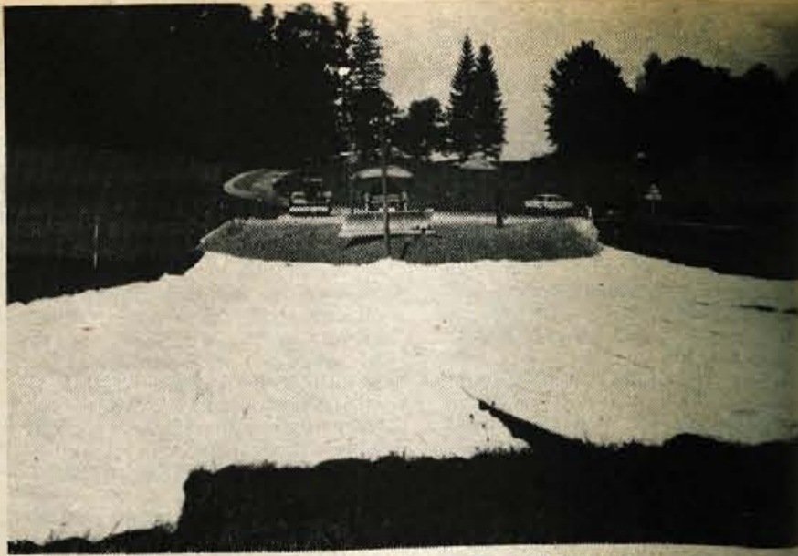
ZACETEK NA CESTI MED GORIČAMI IN GOLNIKOM – Cestno podjetje iz Kranja se je lotilo pripravljajnih del za rekonstrukcijo ceste med Goričami in Golnikom. Na nekaterih odsekih nove trase so podlago že položili posebno maso, ki se je izkazala že pri gradnji na podlagi ceste proti Goričam kot dober preprečevalec vdora vlage v podlago pod cestiščem. Nanjo so že navozili gramoz, ki se bo čez zimo ustalo. Glavna dela na tej cesti pa se bodo začela prihodnje leto. (jk) – Foto: F. Perdan
