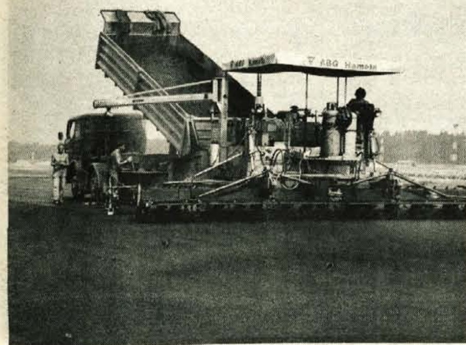
Orjaški finišeji so na brniškem letališču dnevno vgradili na vzlet-nopristajalno stezo nad 4000 ton asfalta – Foto: F. Perdan
