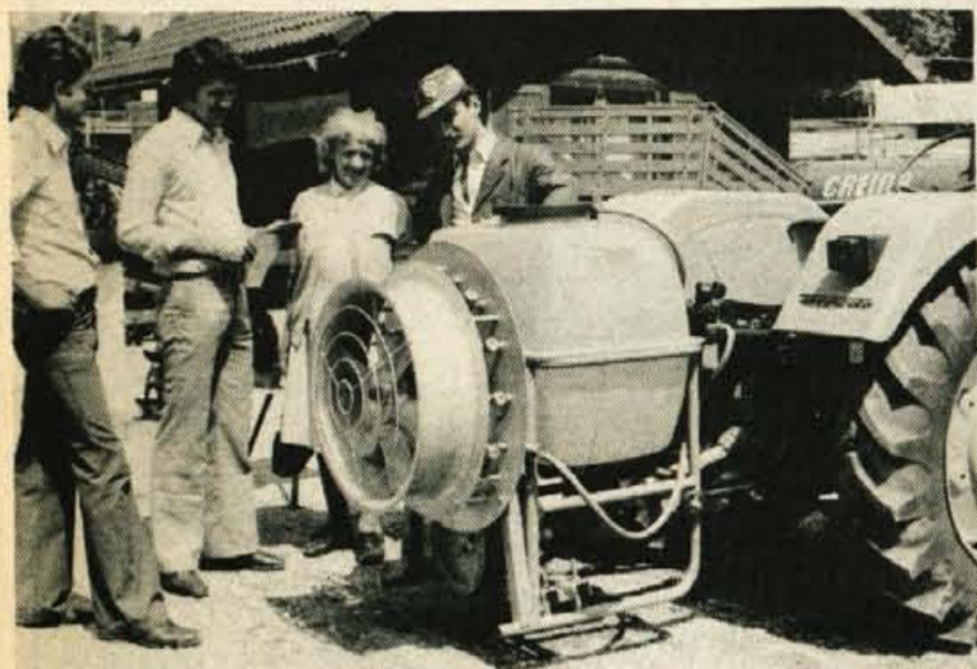
Pri KŽK je največ zanimanja za ATOMIZER, stroj za škropljenje vinogradov in sadovnjakov. Spomladi so ga prvič predstavili na demonstraciji v Ormožu, pravijo pa, da bodo tudi na sejmu imeli z njim vsak dan demonstracije. Je pa standardiziran in se da priključiti na vsak traktor.
