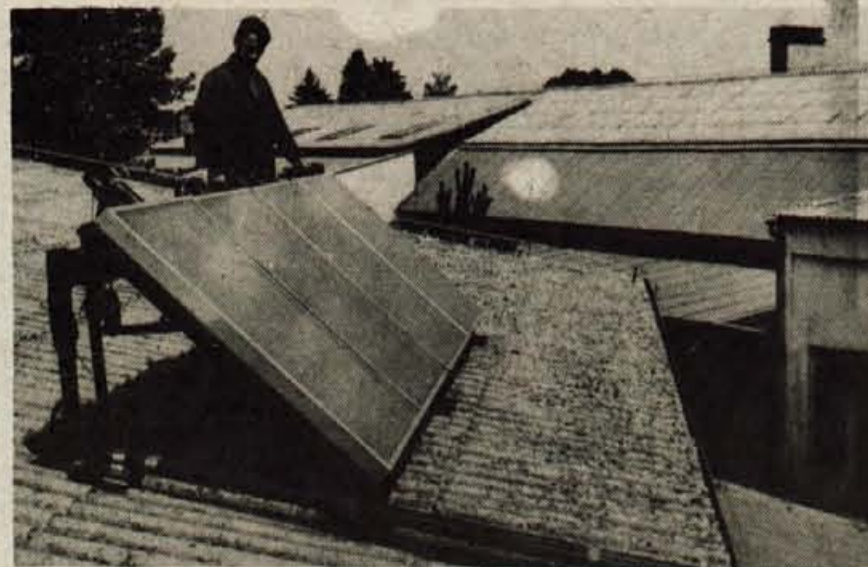
Stirje sončni kolektorji na strehi Zavoda za hlajenje in klimatizacijo na Trati pri Škofji Loki bodo omogočili številne praktične raziskave o tem, kako je v naših vremenskih razmerah mogoče uporabljati sončno energijo za ogrevanje vode. — Foto: F. Perdan
