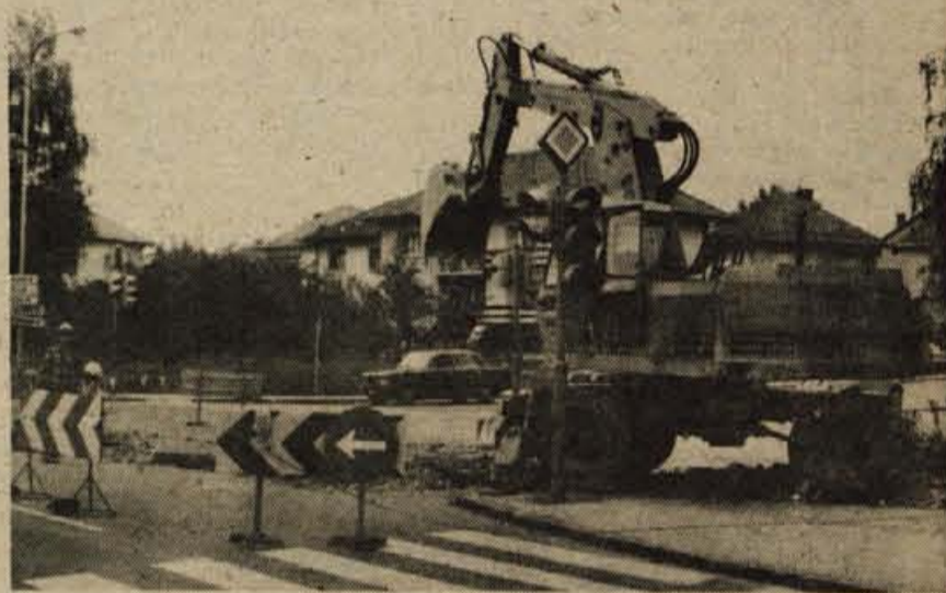
V KRANJU MODERNIZIRAJO KANALIZACIJO - Delavci temeljnih organizacij združenega dela Gradnje pri kranjskem Komunalnem, obrtnem in gradbenem podjetju so začeli pretekli teden rekonstruirati oziroma modernizirati kanalizacijo, ki poteka mimo Dijaškega doma ob obvoznici prot glavnemu kanalu ob Savi. Stara kanalizacija je imela predvsem premajher presek cevi, kar je povzročalo pogoste poplave. V Komunalnem, obrtnem in gradbenem podjetju računajo, da jih čaka na tem področju še za dober teden dela. Financiranje modernizacije kanalizacije je zagotovljeno in urejeno Sredstva so bila načrtovana v skladu za modernizacijo in vzdrževanje kanalizacije v kranjski občini. (jk) - Foto: F. Perdan
