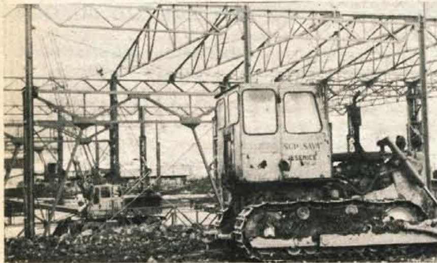
Trgovsko podjetje Universal gradi na Plavškem travniku na Jesenicah veliko tripasovno pokrito skladišče, kjer bo okoli 7.000 kvadratnih metrov prostora. Na severovzhodni strani pa grade tudi novo poslovno zgradbo. Gradbena dela opravljajo delavci SGP Sava Jesenice, konstrukcijo hal pa so izdelali in jih montirajo delavci Metalne iz Maribora. Foto: B. B.
