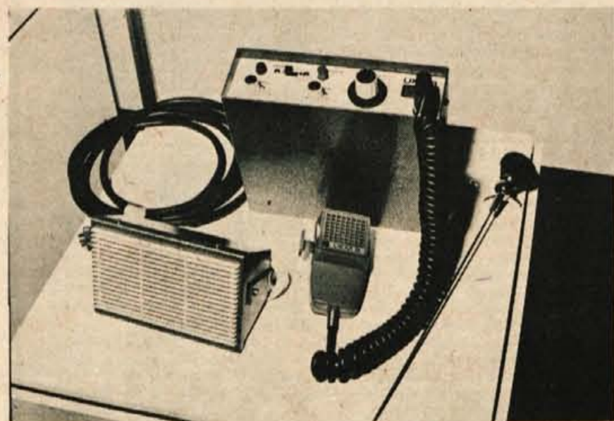
UK-20-TC/6 – Tudi to napravo uporabljajo v civilni zaščiti in ljudski obrambi. Razvili in izdelali so jo v Iskri.
