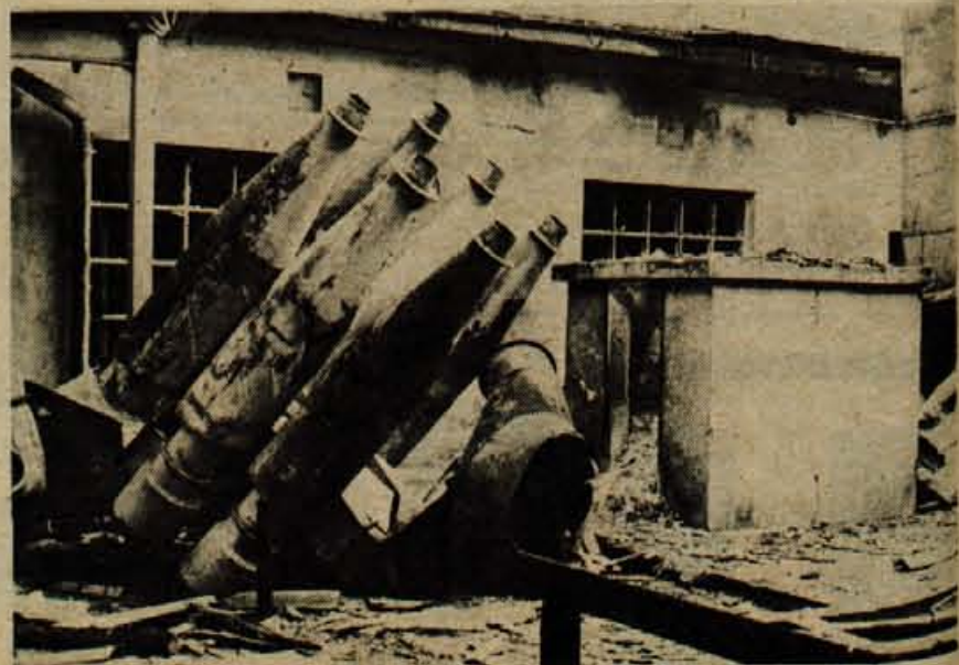
Šestcevni ciklon (na fotografiji) tvori srce prezračevalne naprave, ki jo sestavljata še sistem odvajalnih cevi ter betonski silos. Vžig drobcev v njej je povzročil prašno eksplozijo z znanimi posledicami — Foto: M. K.
