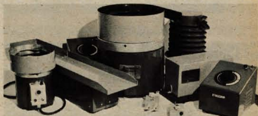
Vibracijski dodajalniki
