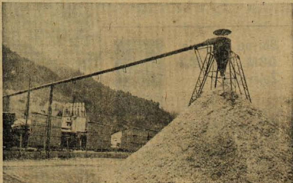
Obrtni center iz Žirov za žago Slovenjalec v Spodnji Idriji izdelal moderno napravo za transport lesnih odpadkov
