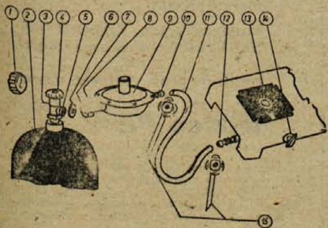
1. varnostna matica, 2. jeklenka, 3. ventil jeklenke, 4. vreteno ventila, 5. ustje ventila, 6. tesnilka, 7. nastavek regulatorja, 8. matica regulatorja, 9. regulator, 10. nastavek za gumijasto cev na regulatorju, 11. gumijasta cev, 12. nastavek za gumijasto cev na aparatu, 13. gorilna krona, 14. gumb plinskega aparata, 15. objemki
