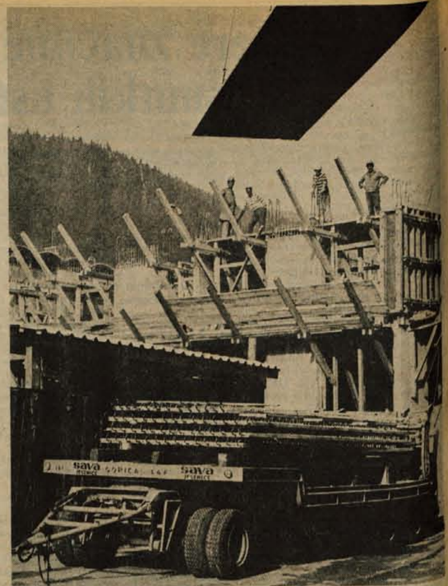
Nova tehnologija omnia plošč in litega betona omogoča gradbenemu podjetju Sava, da gradi največjo stolpnico na Gorenjskem hitreje in ceneje. Gradnja poteka po montažnem programu.
