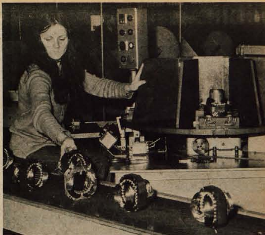
Pred štirinajstimi dnevi so v Iskri namestili nov stroj za električno navijanje žic za statorje elektromotorčkov. Izdelali so ga po zamisli domačih strokovnjakov — Foto: F. Perdan
