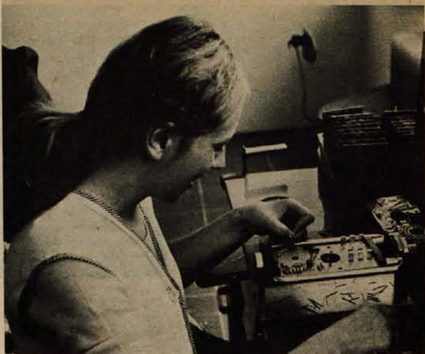
Spajkanje osnovne plošče pri univerzalnem instrumentu US 7 a.
