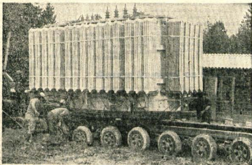
Podjetje Hidromontaža Maribor je pripeljalo v četrtek v Kranj transformator za novo razdelilno transformatorsko postajo na Laborah, ki bo začela obratovati letošnjo jesen. Transformator, ki so ga v četrtek pripeljali v Kranj, tehta 59 ton. (Jk) — Foto: F. Perdan
