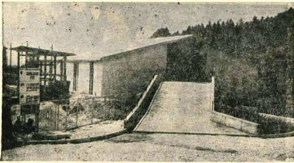
Splošno gradbeno podjetje Projekt iz Kranja je zgradilo v novem stanovanjskem naselju na Bistrici pri Trliču garaže. Prvi objekt ki ga prikazuje naša fotografija, je že zgrajen. V njem dva prostora za 60 avtomobilov. Ena garaža stane 13.000 dinarjev. Projekt namerava zgraditi še dva podobna objekta takoj, ko bo za nove garaže dovolj zanimanja. (jk) — Foto: F. Perdan
