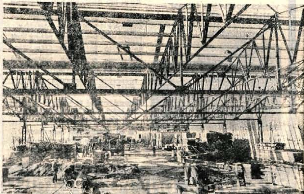
Ob cesti Skofja Loka—Trata gradi podjetje Jelovica okrog 6000 kvadratnih metrov veliko lope za vskladiščenje žaganega lesa. V lopi bodo uredili tudi sušilnice, brusilnice in kompresorsko postajo. Konstrukcijo, ki je na sliki lepo vidna, postavlja podjetje Metalna iz Maribora, gradbena dela izvaja Tehnik Skofja Loka, notranja opravila, napeljava in podobno pa so prevzela številna druga manjša slovenska podjetja (-ig) — Foto: F. Perdan
