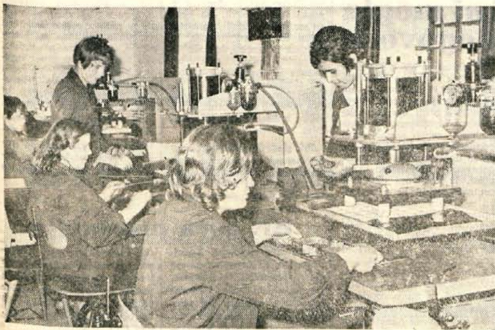
Pogled v enega izmed obratov podjetja Termopol: delavki na visokofrekvenčnem stroju varjata PVC material
