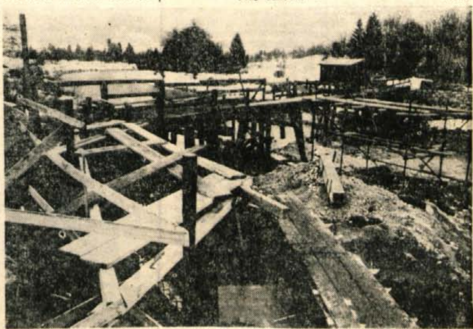
Pri vasi Broč v Bohinjju gradijo čez Savo Bohinjko nov most z betonskimi nosilci. Starega, lesenega, je narasla voda večkrat odnesla, vsa popravila pa so bila samo začasna — Foto F. Perdan
