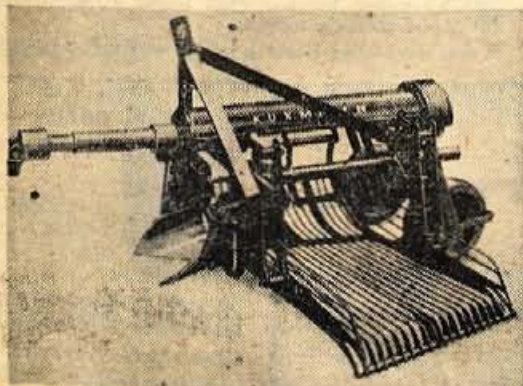
KUXMANN — izkopalnik za krompir
