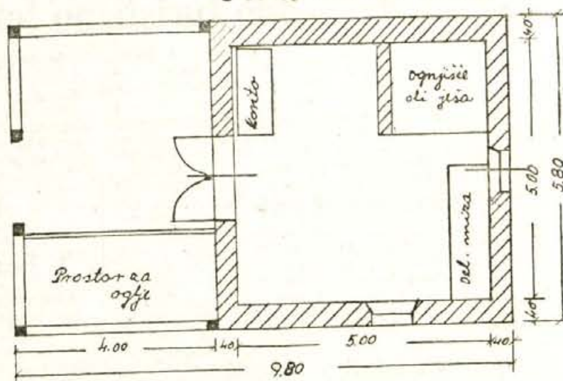
Floris fužine M: 1:100
