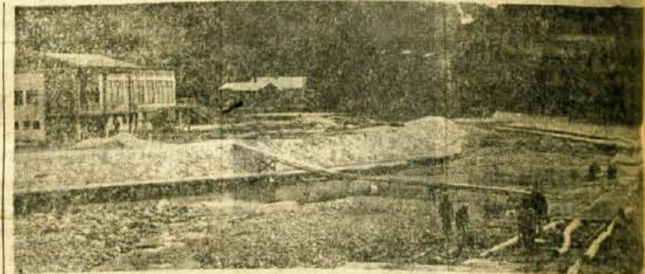
Zadnje poplave so skoraj popolnoma uničile jez na kopalšču v Škofji Loki. Te dni urejajo nov jez. Narediti ga bodo morali v dolžini okoli 45 m, za kar bodo potrebovali 15 milijonov dinarjev. Investicija je velika, vendar bo s tem dokončno rešen problem, saj bo ves jez iz cementsa ter prevlečen z leseno oblogo
