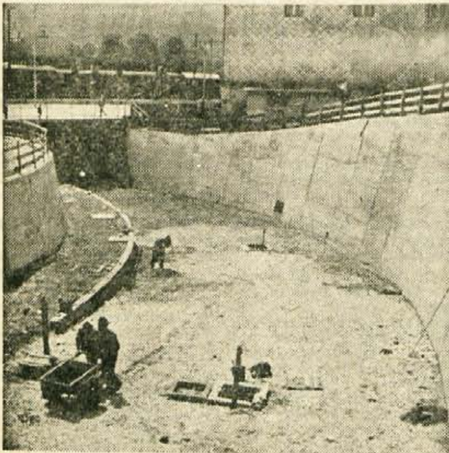
Za ureditev železniškega in cestnega prometa na Jesenicah bo precej pripomogel tudi podvoz, ki ga gradijo poleg Korotana. Le žal, da se ta dela hudo zavlačujejo
