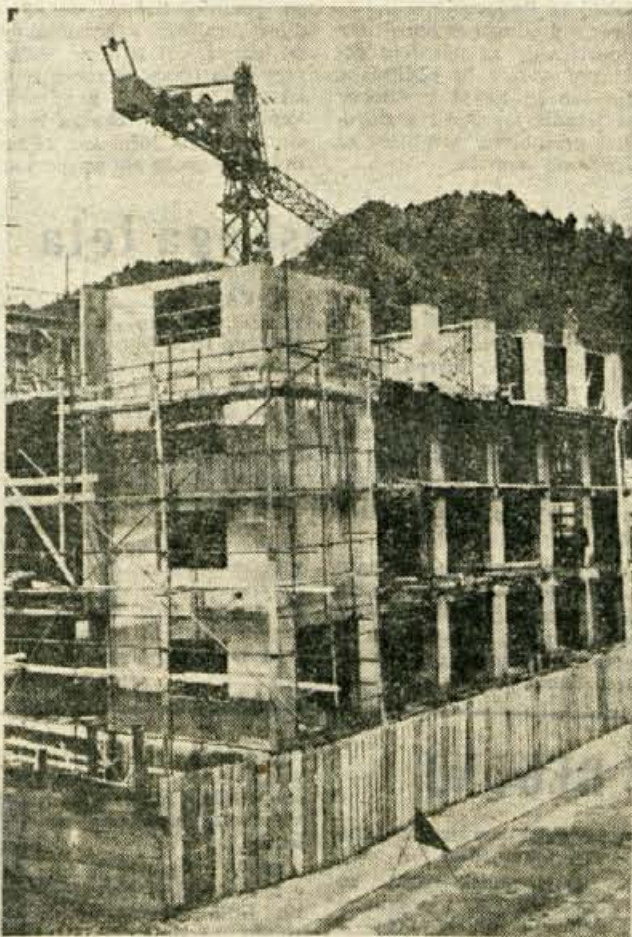
Gradnja 10-nadstropne stolpnice s 56 stanovanji v Trziču je v polnem zamahu. Celotni stroški so predvideni na 300 milijonov dinarjev, prve družine pa se bodo vselile konec prihodnjega leta
