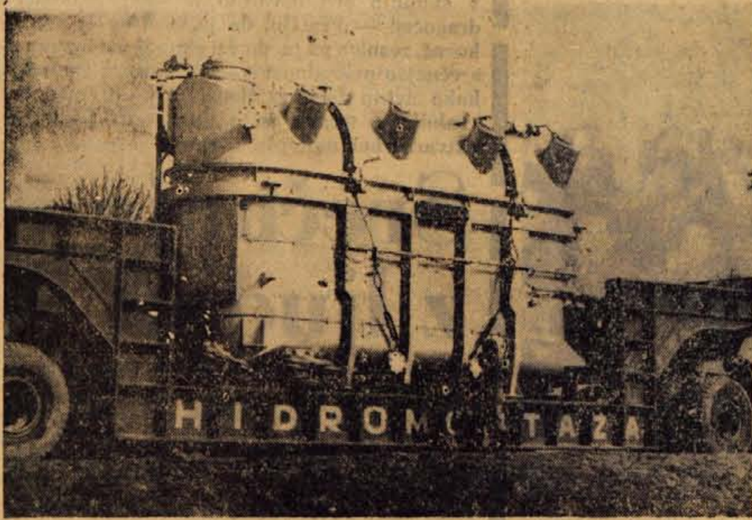
Pred dnevi so v Zirovnicu pripeljali 76 ton težak transformator, ki ga bodo montirali v tamkašnji hidrocentrali. Hidrocentrala se namreč pripravlja na povečanje zmogljivosti, ki jo zahteva povečana produkcija v Zelenarni. Transformator so do Zirovnic pripeljali z vlakom, od proge pa so ga s specialnim vozilom več dni postopoma spravljali do elektrarne
